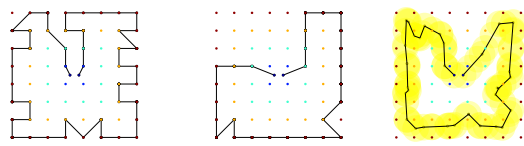
T_{max}=95, \delta=0.0, R=1335 T_{max}=60, \delta=0.0, R=845 T_{max}=60, \delta=1.5, R=1600
