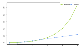
fibonacci-n10.pdf
