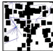
RABIT*
