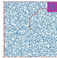
RRT, n=10000
