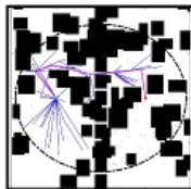
BIT*
