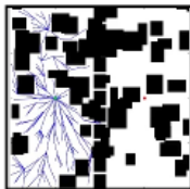
RRT*
