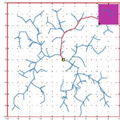
RRT*, n=250
