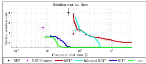
RRT*
