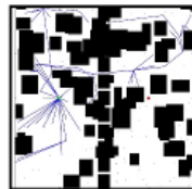
RABIT*
