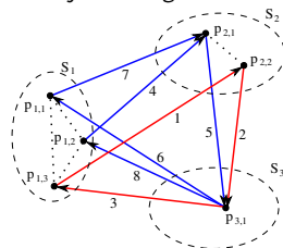
GATSP
