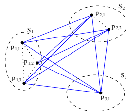
GTSP
