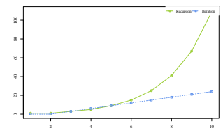
fibonacci-n10.pdf
