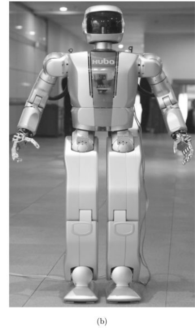
Fig. 1. A Hubo KHR-4 Humanoid Robot.
