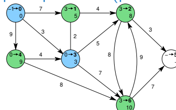
1: Po 2. expanzi má uzel 3 již nejkratší cestu.
