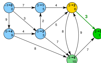
3: Expanzí uzlu 2 získáme cestu též do uzlu 5.
